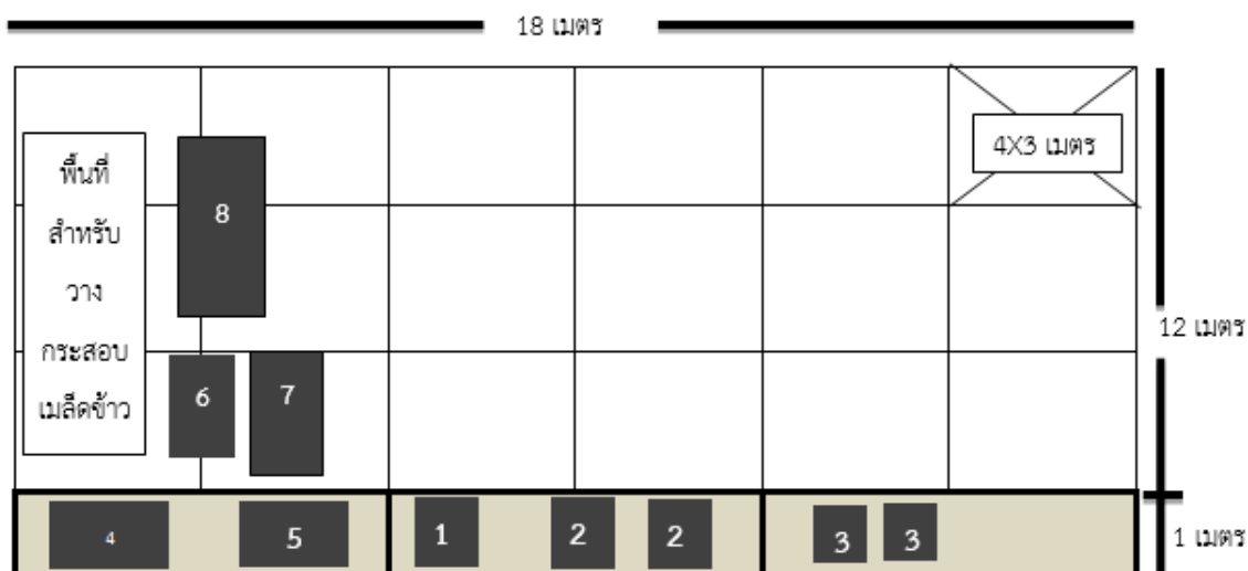
ภาพที่ 3 รูปแบบการวางผังโรงสีแบบที่ 1
