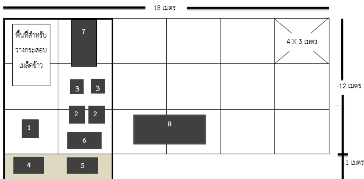
ภาพที่ 4 รูปแบบการวางผังโรงสีแบบที่ 2
